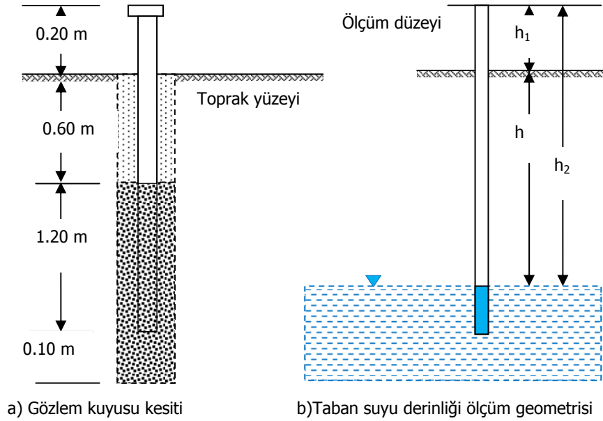
Şekil 2. Gözlem kuyusu kesiti (a) ve taban suyu düzeyi ölçüm geometrisi (b)
