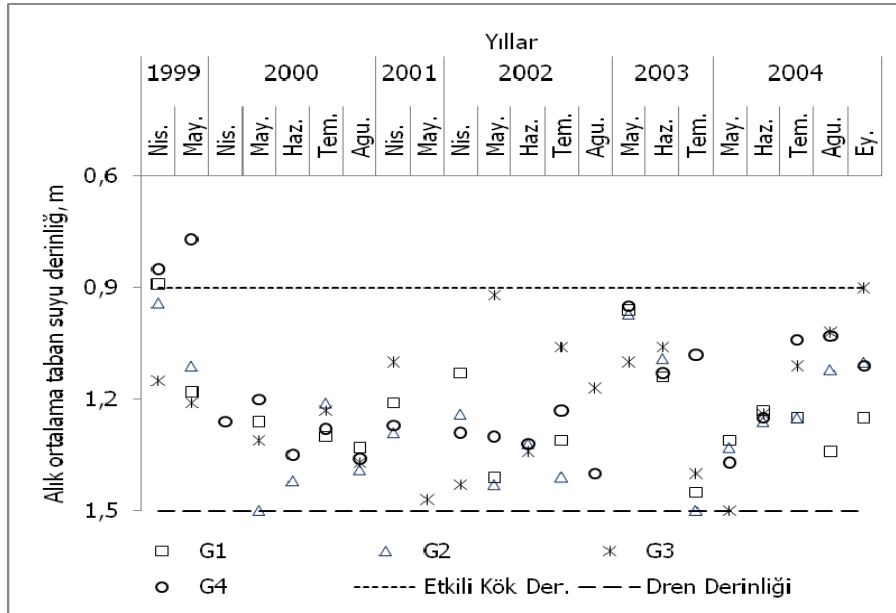
Şekil 4. Aylık ortalama taban suyu derinlikleri
